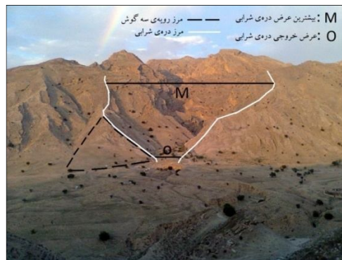
شکل ۹: نحوه اندازه‌گیری پارامترهای شاخص دره‌های ساغری
