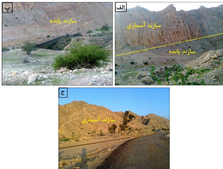
شکل ۵: الف) مرز سازندهای آسماری و پایه در water gap اصلی تاقدیس، ب) رخنمون سازند پایه در water gap، ج) نمایی از رخنمون سازند آسماری در یال جنوب غربی تاقدیس خويز
