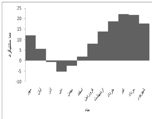
شکل ۴: مقادیر دمای ماهانه و سالانه (برحسب سانتی گراد) در ایستگاه کوهرنگ
