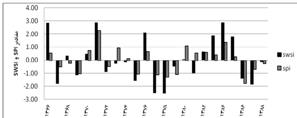
شکل ۱۰: مقایسه مقادیر SPI و SWSI سالانه حوضه سد زاینده رود
