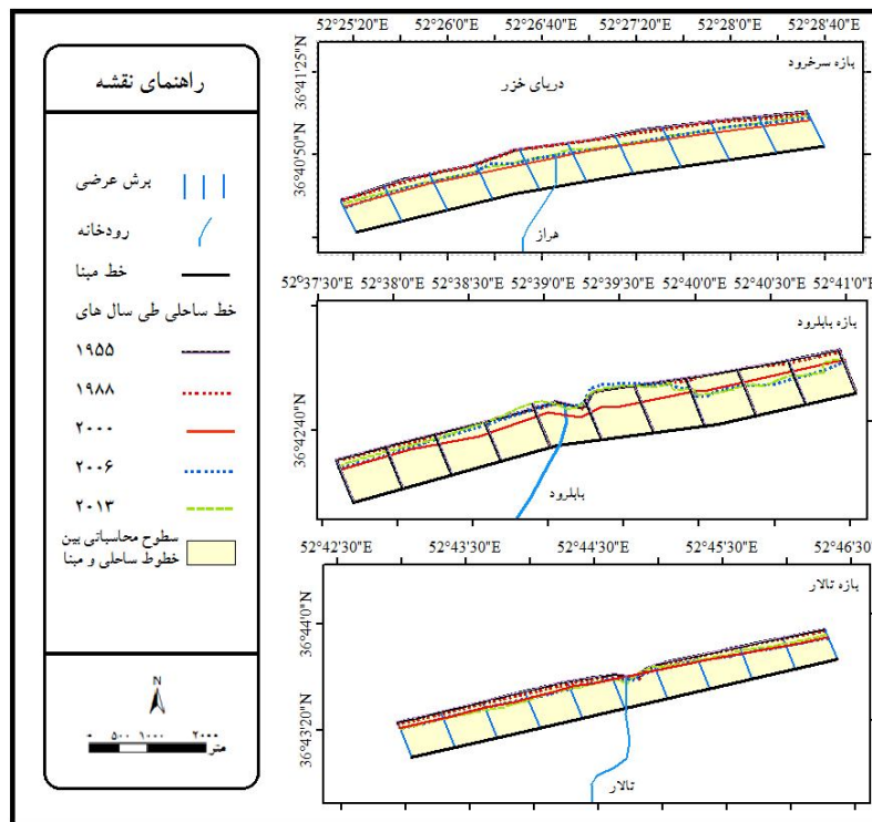
شکل ۳: نقشه تغییرات خط ساحلی طی سال‌های ۱۹۵۵-۲۰۱۳
