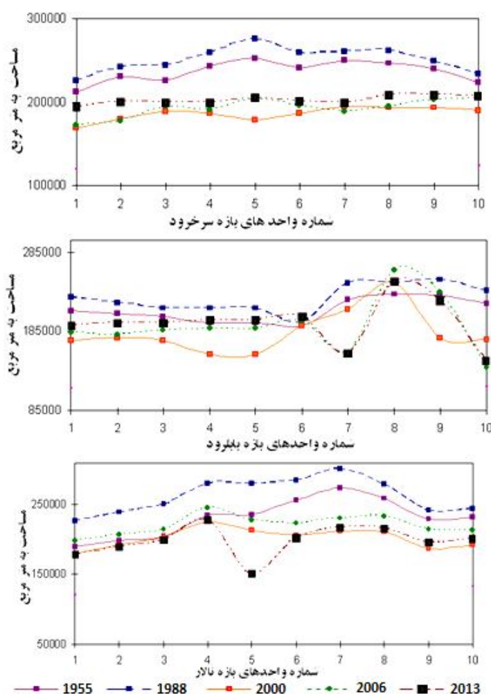
شکل ۱۱: تغییرات مساحت در واحدهای ده‌گانه بازه‌های رودخانه‌ای سرخ‌رود، بابل‌رود و تالار
