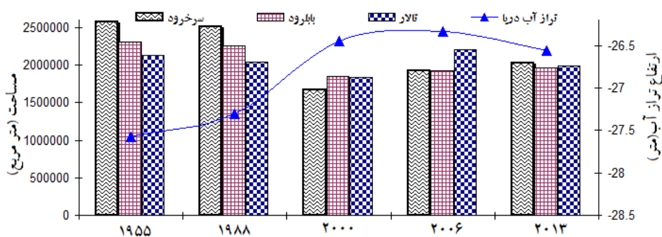
شکل ۶: ارتباط مساحت بازه‌ها و تراز سطح آب دریا
