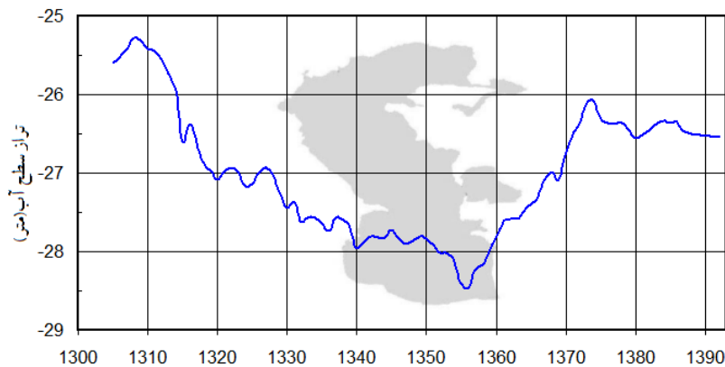
شکل ۵: نوسان سطح آب دریای خزر در ایستگاه ترازسنجی انزلی، طی سال‌های ۱۳۰۸-۱۳۹۲.
