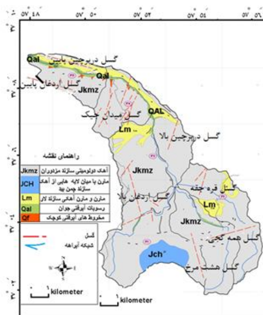
شکل ۲: نقشه زمین شناسی حوضه مورد مطالعه (منبع: نقشه زمین شناسی شیروان مقیاس ۱:۱۰۰۰۰۰)
