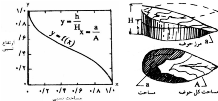
شکل ۲: منحنی هیپسومتری بی بعد
