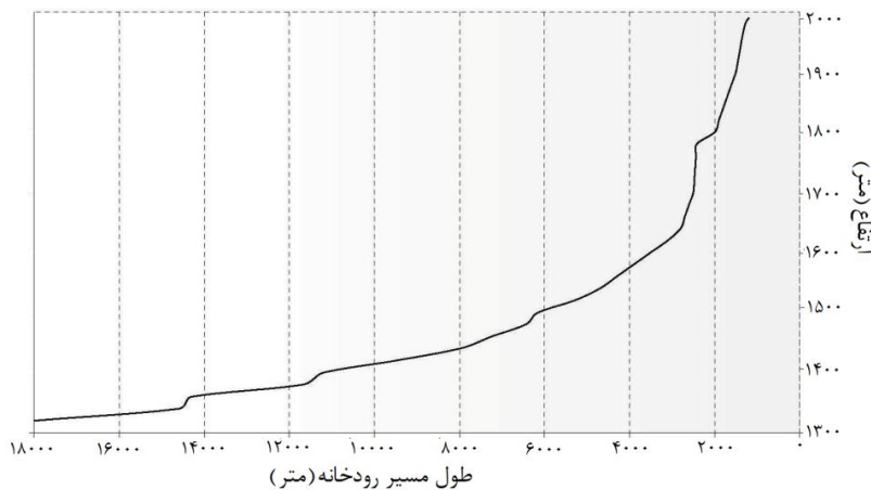
شکل ۳: پروفیل طولی رودخانه قزلچه سو در حوضه مورد مطالعه
